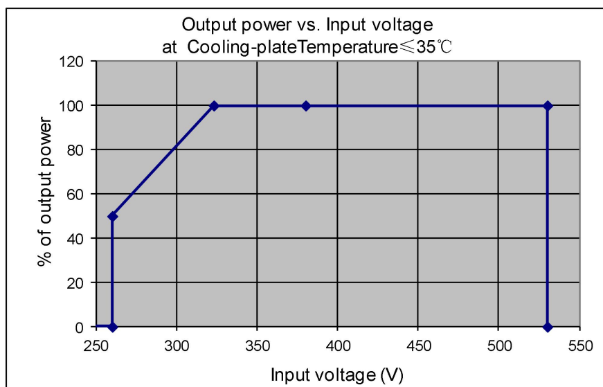
图 4.1 输入限功率曲线
